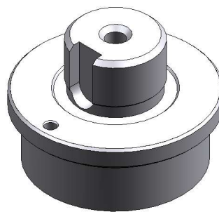
500/3DP Punzone per diametri con 1 chiavetta per la versione originale e 2 per la versione tipo BMT
