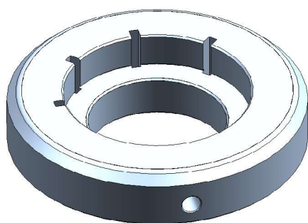
600/5M Adattatore per matrici da stazione originale a stazione 70 mm
