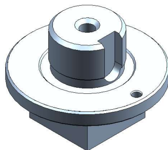
500/3SP Punzone per sagomati con 1 chiavetta per la versione originale e 2 per la versione tipo BMT
